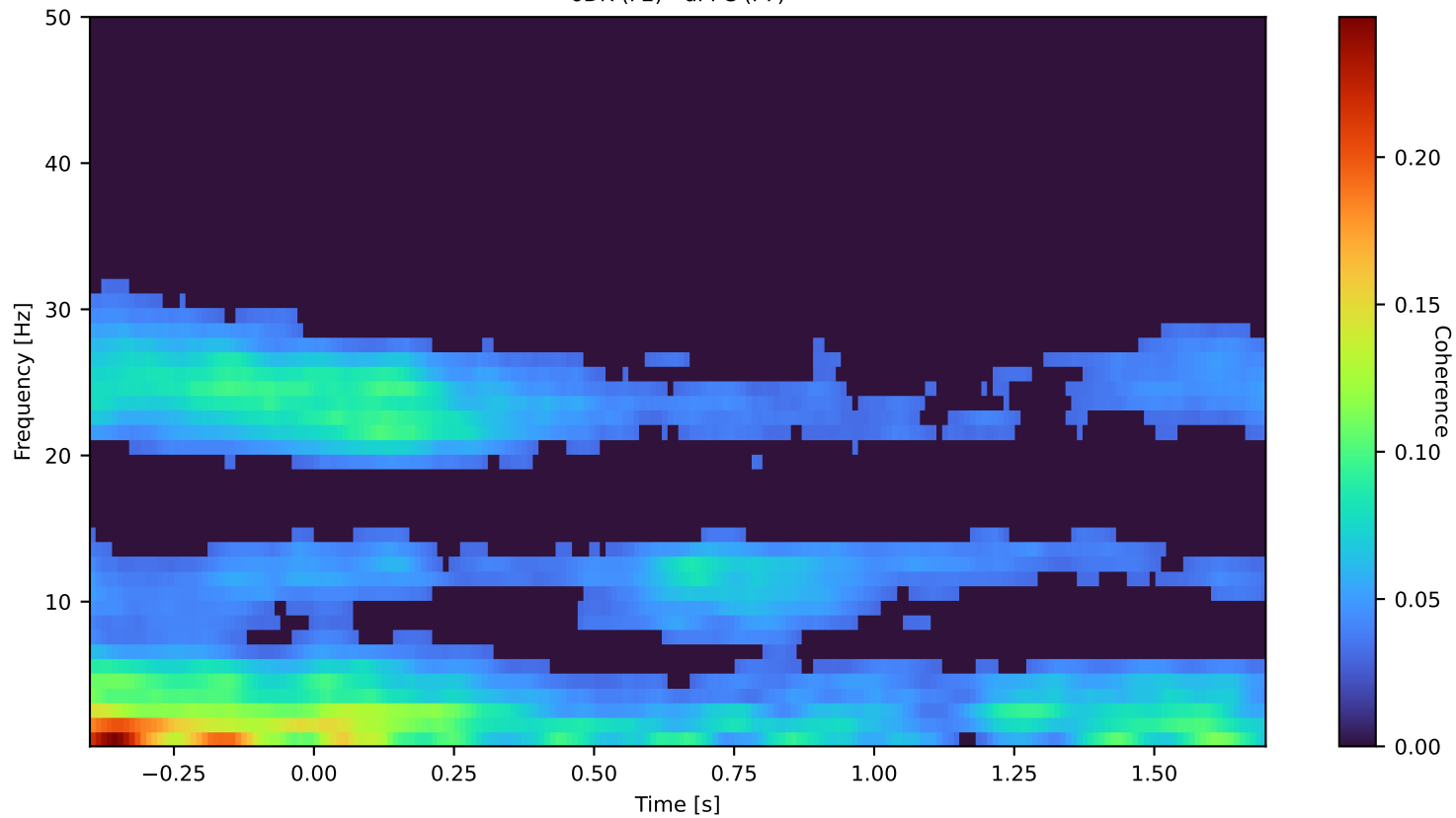
6DR (F2) - dPFC (F7)
